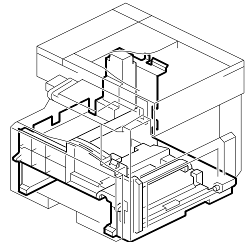
18. FRAME SECTION
